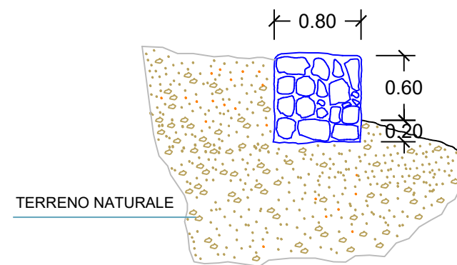
SEZIONE MURI n. 3 e 4
