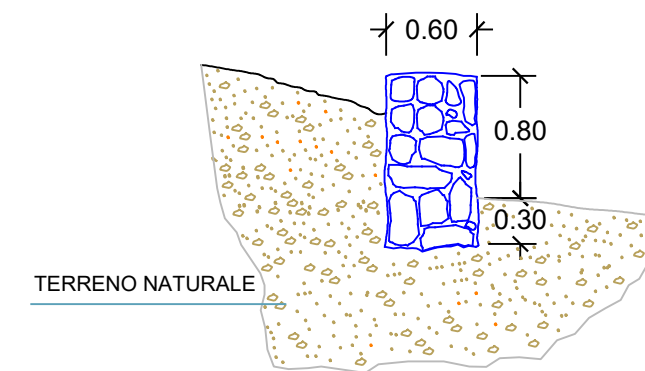
SEZIONE MURO n. 6
