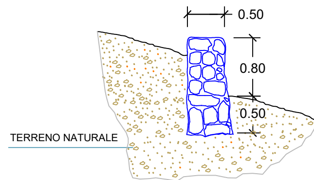
SEZIONE MURO n. 1
